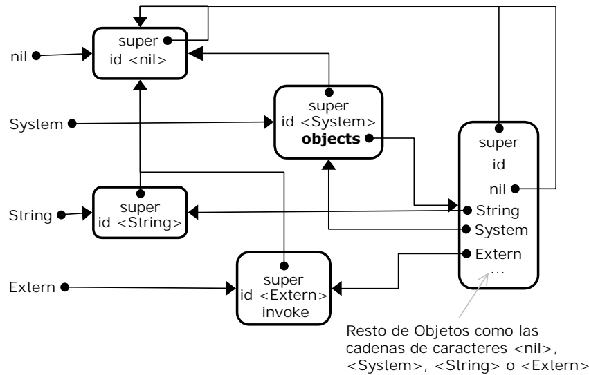
Figura 12.3: Acceso a los objetos de la máquina abstracta mediante el objeto “System”.
