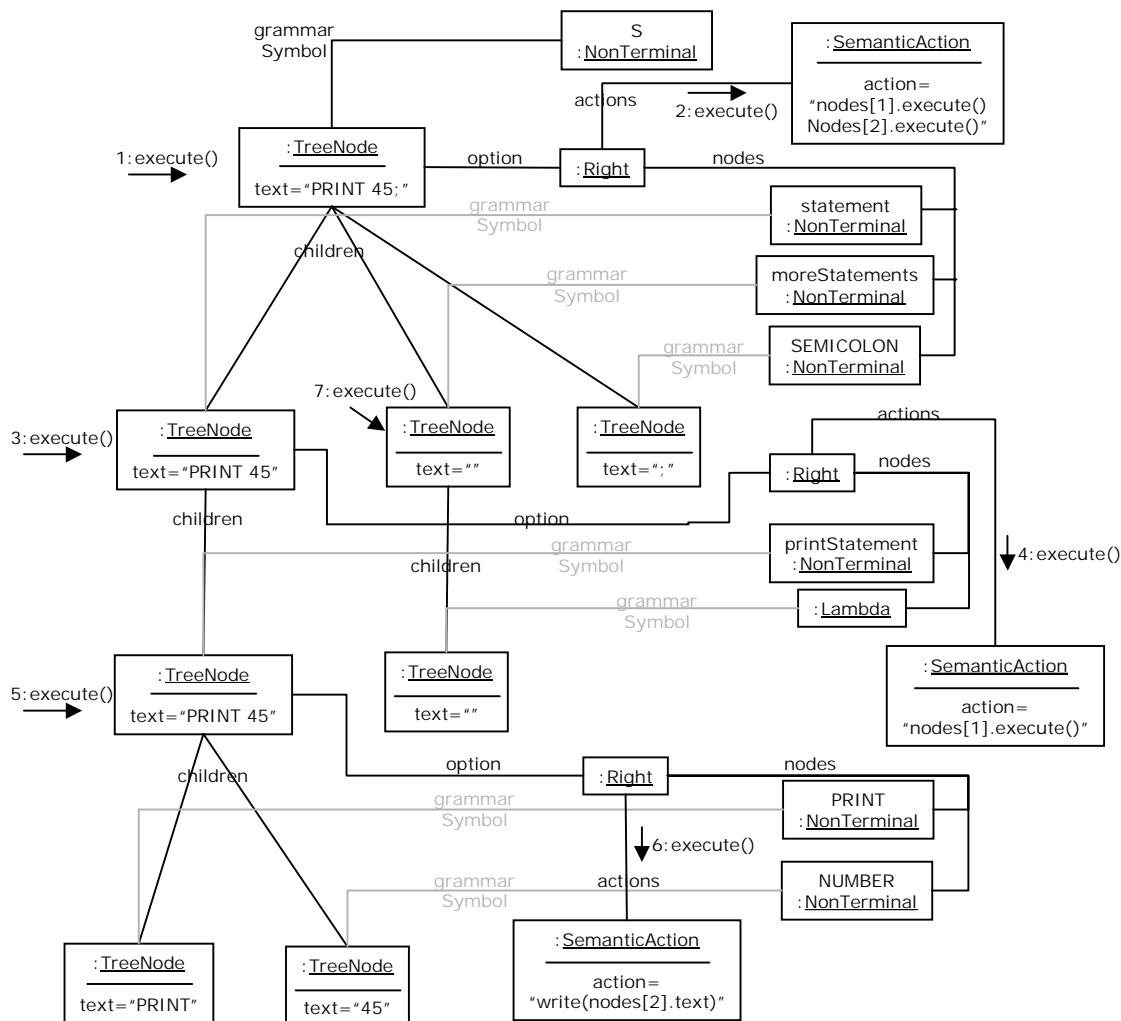
Figura 14.9: Evaluación de un árbol sintáctico.
