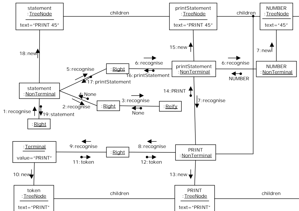
Figura 14.7: Creación del subárbol sintáctico propio de una sentencia.
